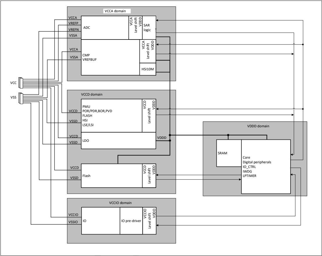
图 2-2 电源框图
