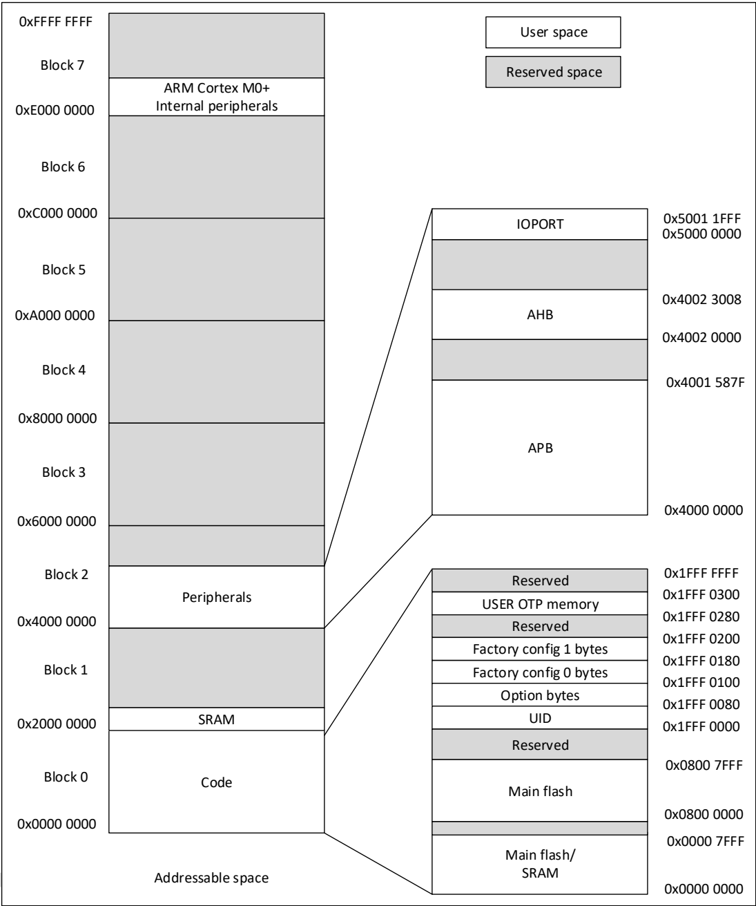
图 4-1 存储器映射
