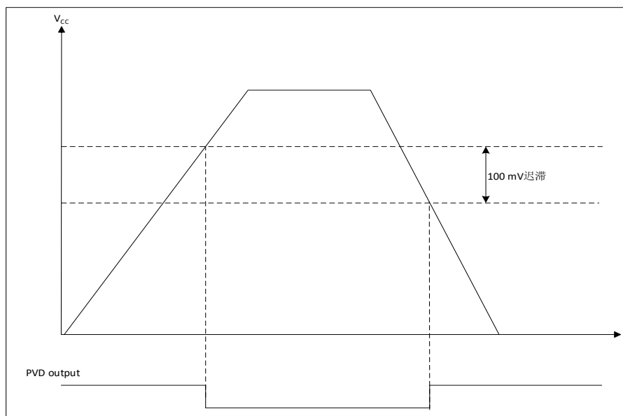
图 2-4 PVD 阈值
