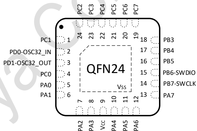
图 3-2 QFN24 Pinout1 PY32CA80E1xU7 (Top view)
