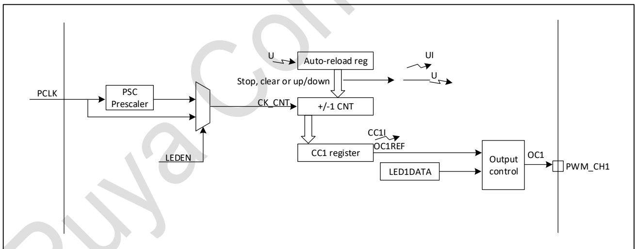
图 15-1 PWM 模块框图
