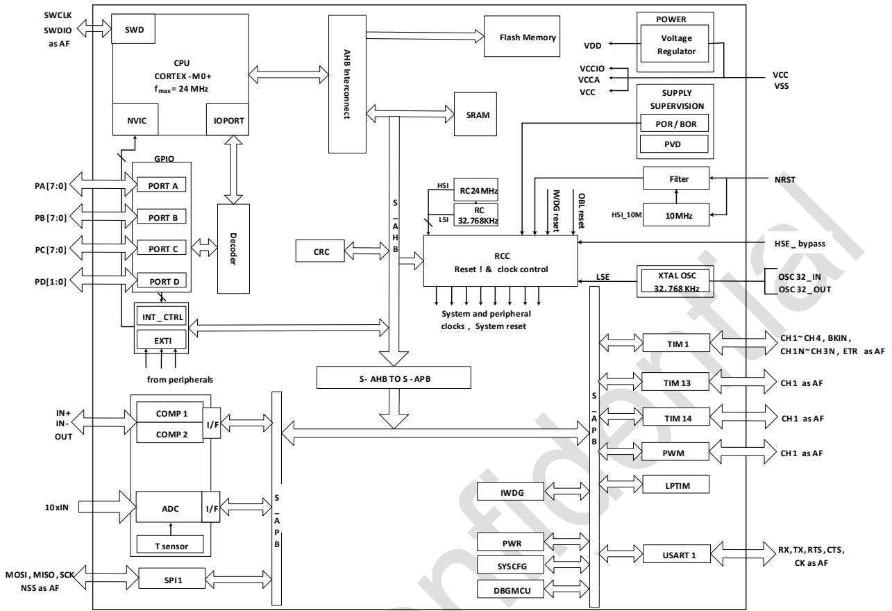
图 2-1 系统架构框图
