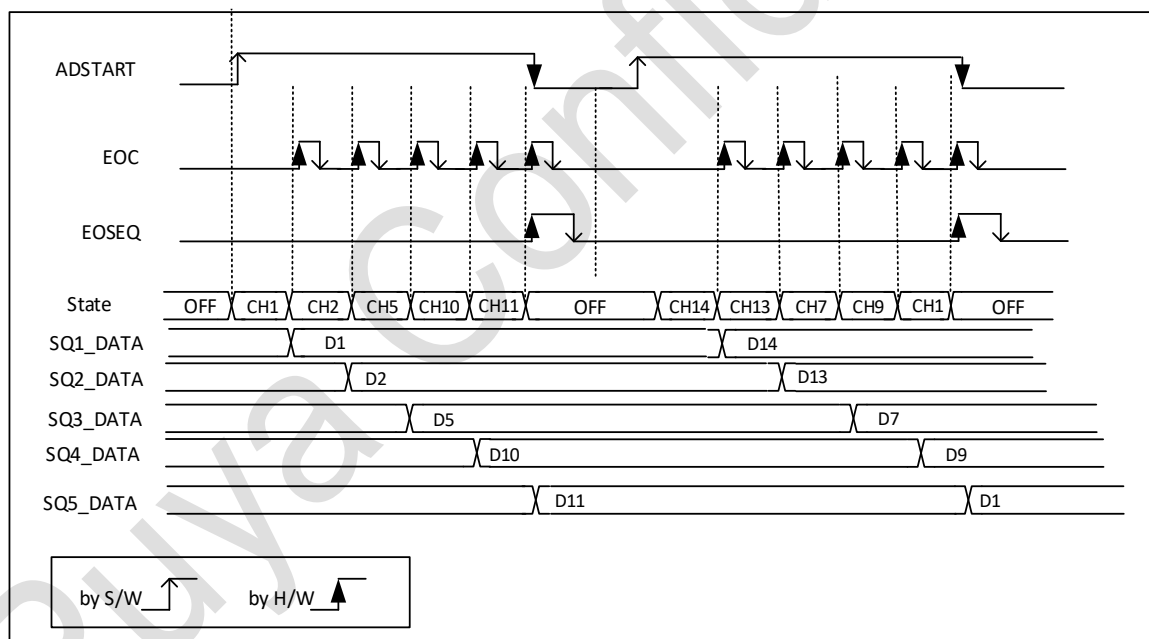
图 11-7 序列的单个转换, 软件触发
