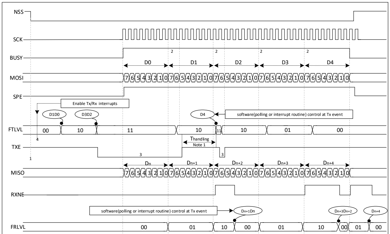
图 19-10 主机全双工通信图(bit frame=8)
