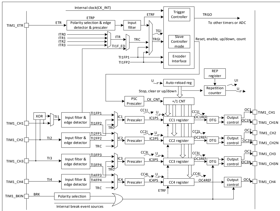
图 13-1 高级控制定时器架构框图
