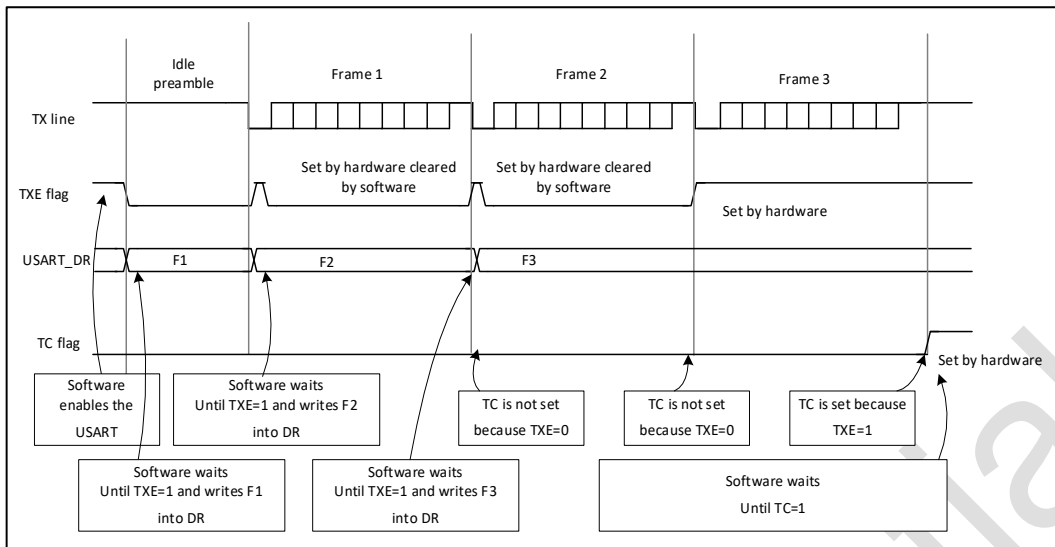
图 18-4 传输时 TC/TXE 的时序
