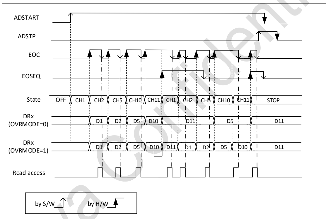
图 11-11 过载
