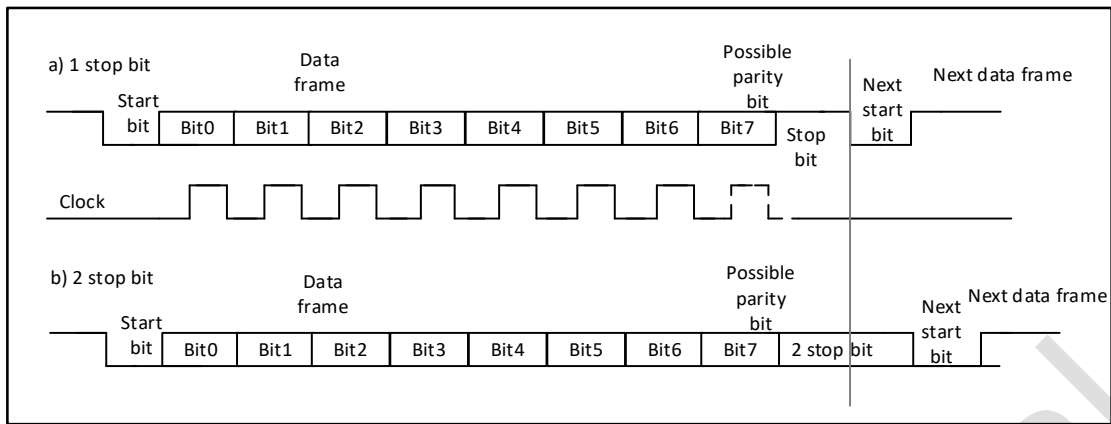
图 18-3 配置停止位
