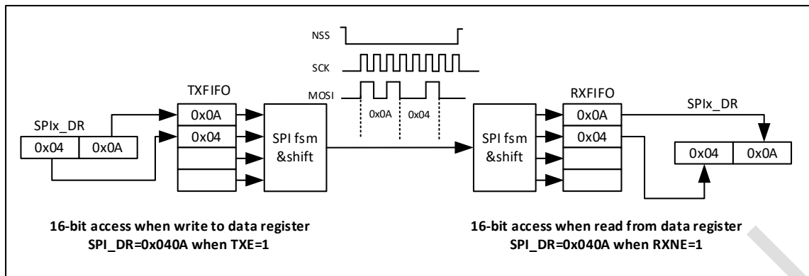
图 19-9 FIFO 中的数据包传输与接收
