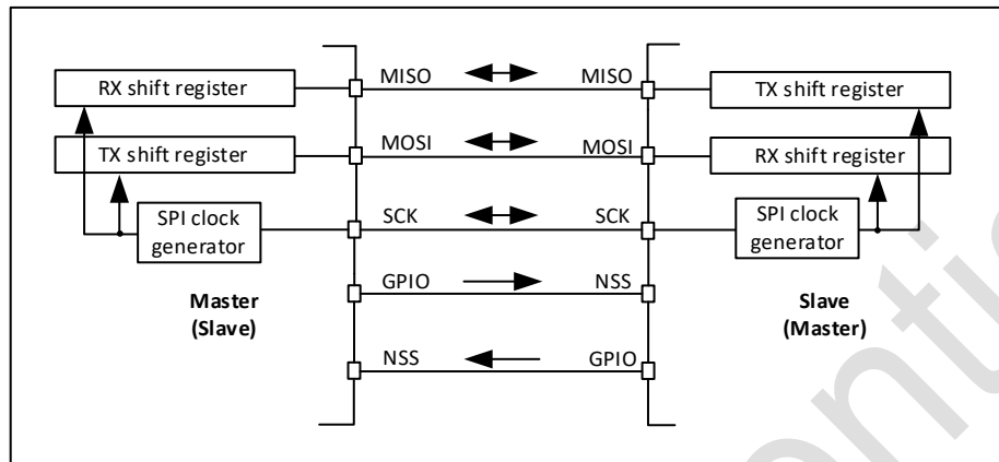
图 19-6 多主机应用
