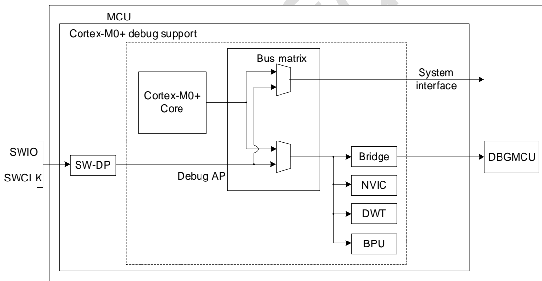
图 21-1 DBG 框图
