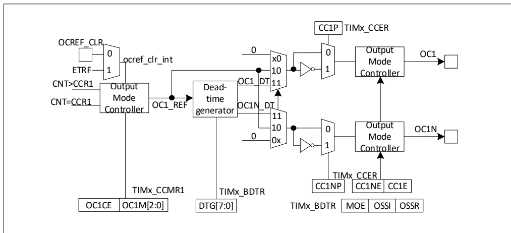
图 13-29 捕获/比较通道的输出部分(通道 1 至 3)
