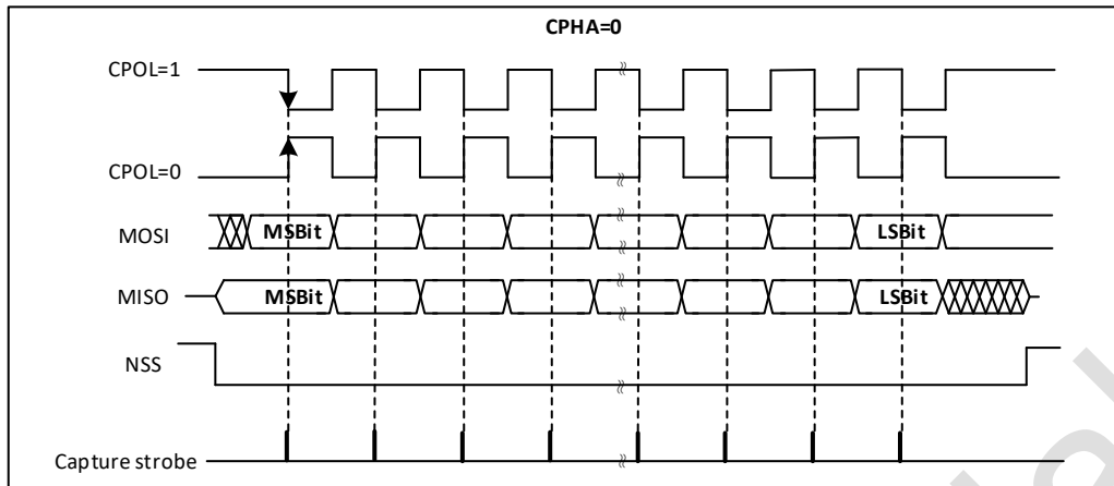
图 19-8 数据时钟时序图
