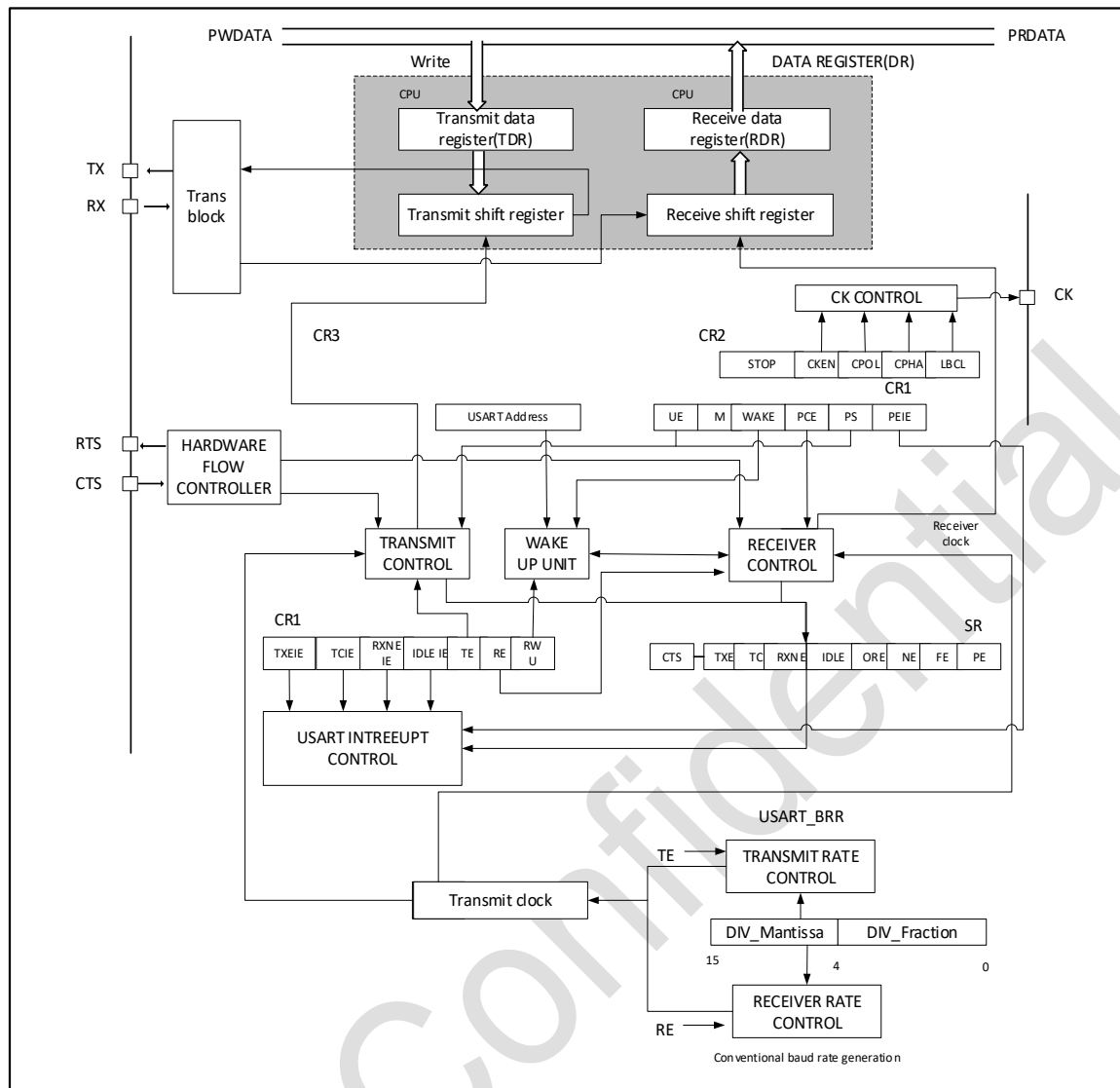
图 18-1 USART 框图
