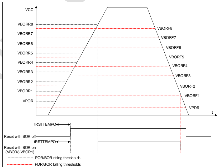
图 5-2 POR/PDR/BOR 阈值
