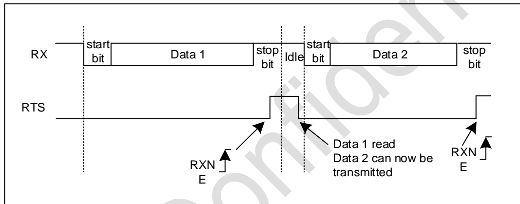
图 18-14 RTS 流控制
