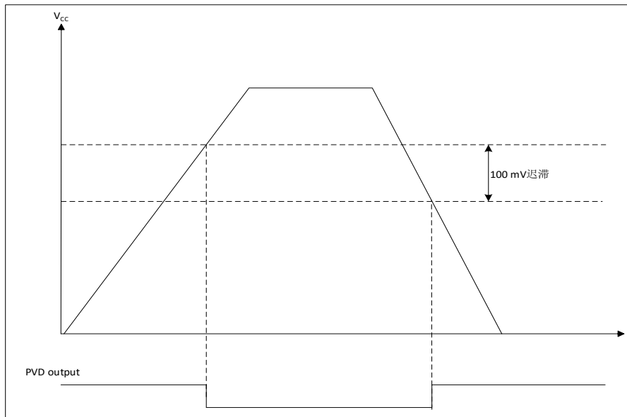
图 5-3 PVD 阈值
