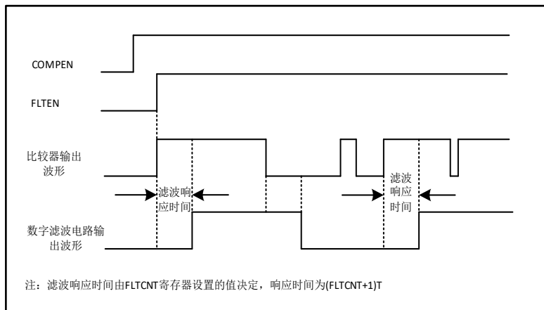
图 12-3 COMP 滤波
