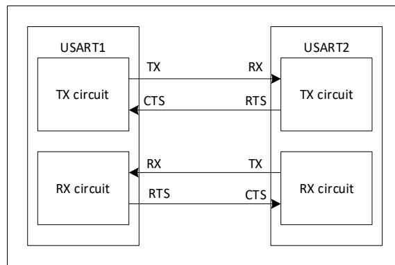
图 18-13 两个 USART 间的硬件流控制
