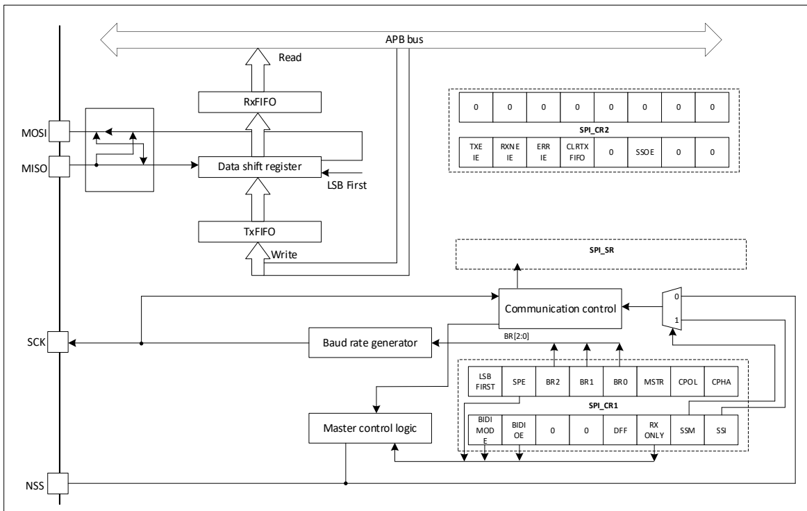
图 19-1 SPI 框图
