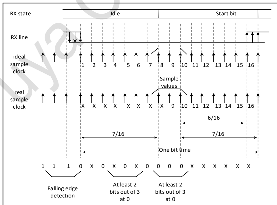
图 18-5 开始位检测
