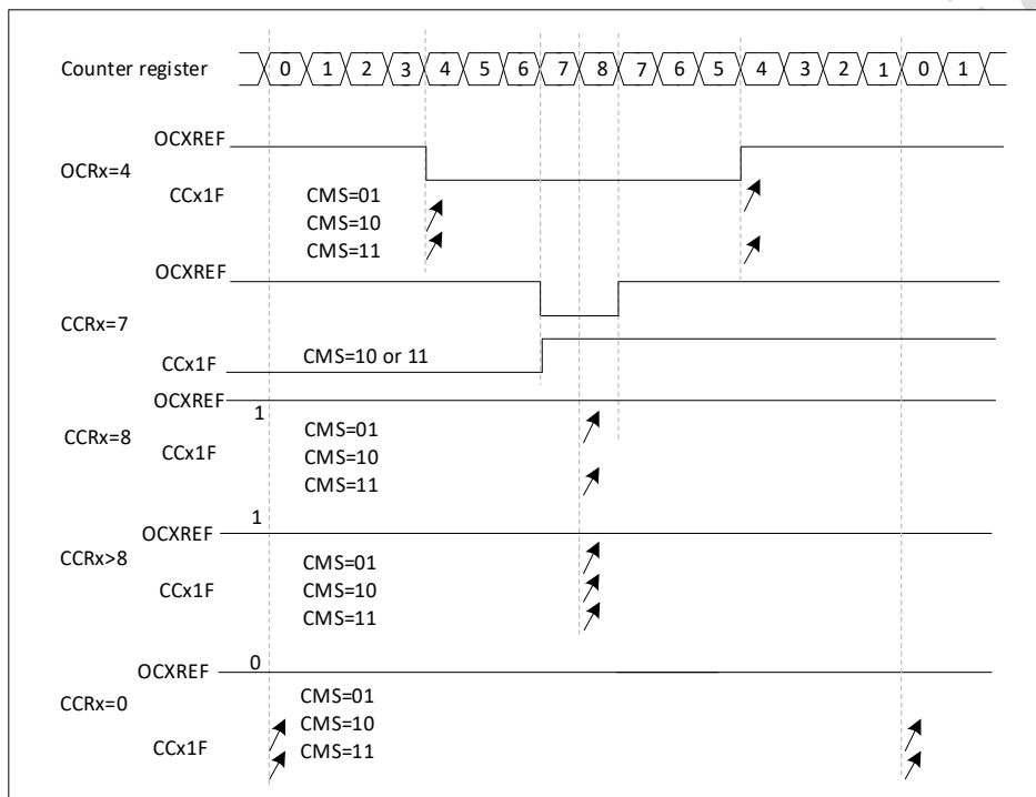
图 13-34 中央对齐的 PWM 波形(APR=8)
