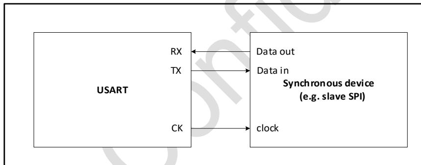
图 18-9 USART 同步传输的例子
