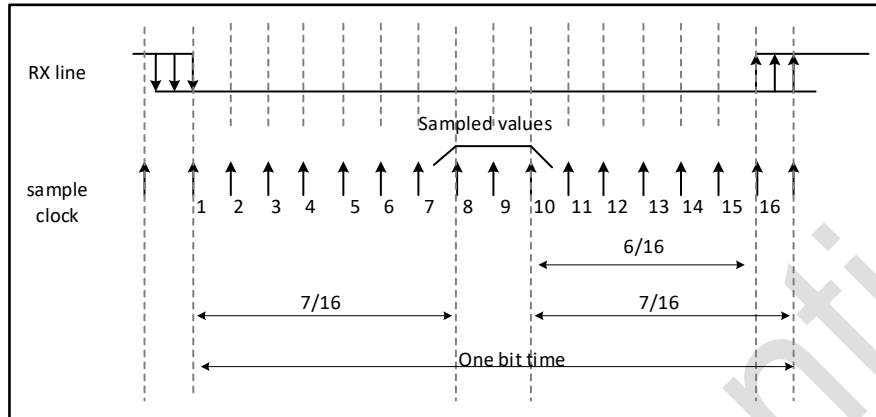
图 18-6 检测噪声的数据采样
