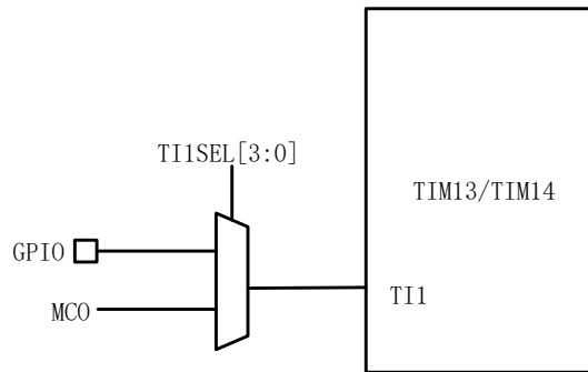
图 6-3 频率测量与 TIM14 捕获模式
