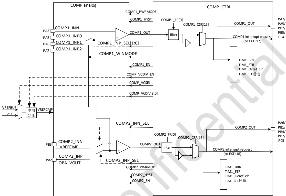
图 12-1 比较器架构框图
