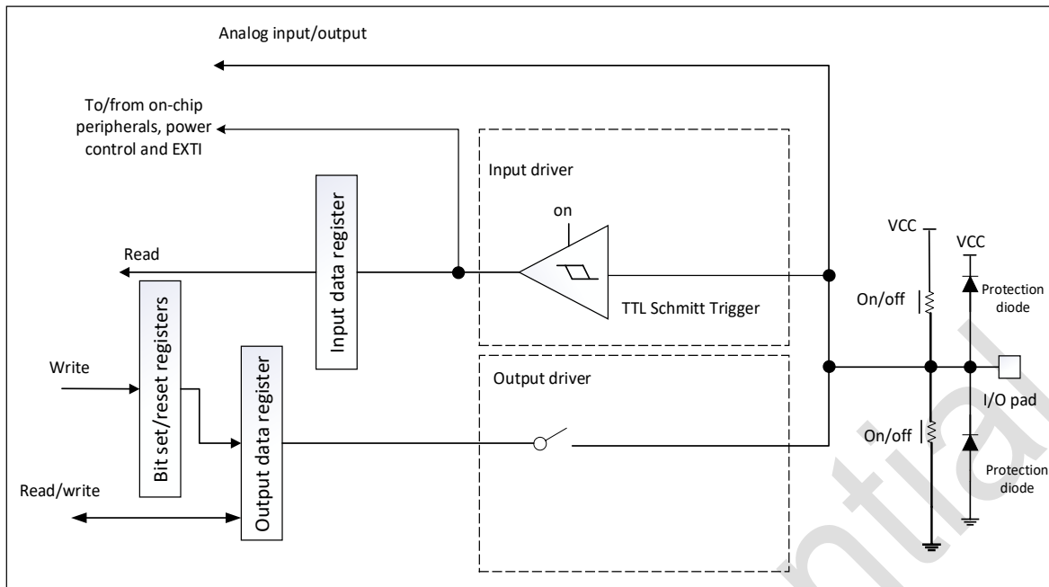
图 7-2 输入浮空/上拉/下拉配置
