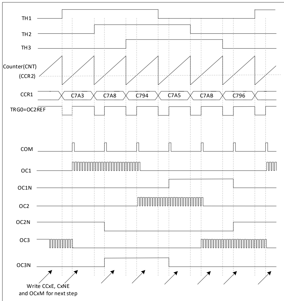
图 13-47 IC1FP1 霍尔传感器接口的实例
