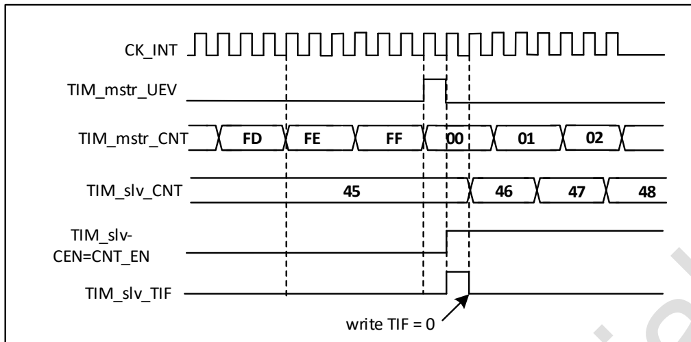
图 13-56 使用 TIM_mstr 的更新触发 TIM_slv
