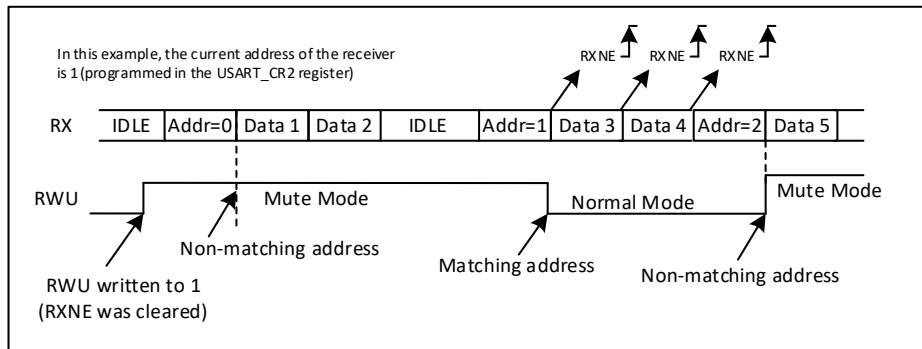
图 18-8 利用地址标记检测的静默模式
