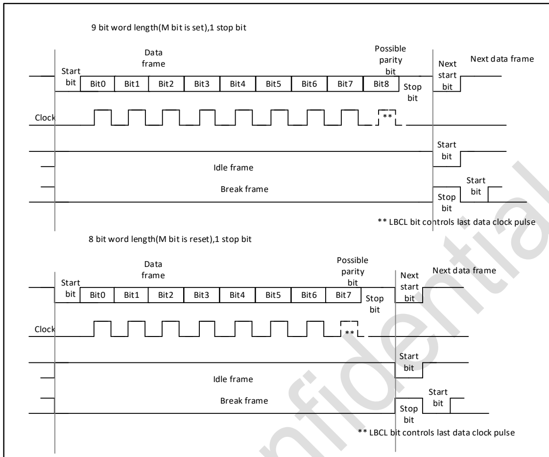
图 18-2 字长设置
