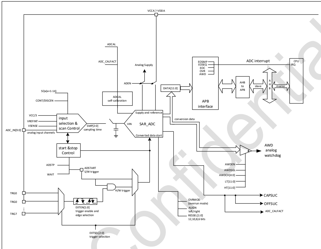
图 11-1 ADC 框图
