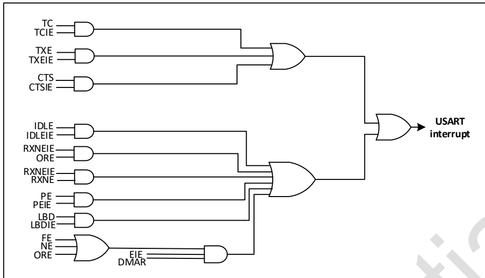
图 18-161 USART 中断映像图
