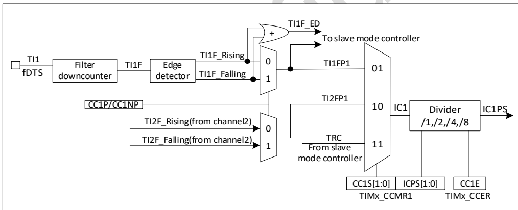
图 13-27 捕获/比较通道(如：通道 1 输入部分)
