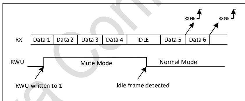
图 18-7 利用空闲总线检测的静默模式
