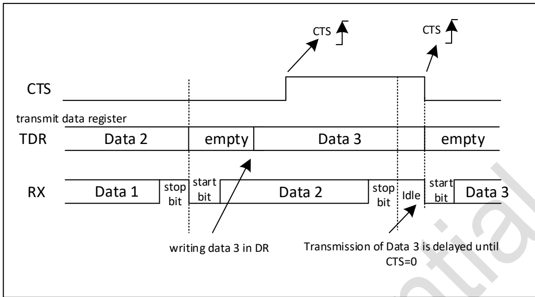
图 18-15 CTS 流控制
