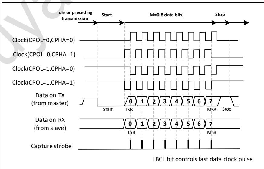
图 18-10 USART 数据时钟时序示例(M=0)
