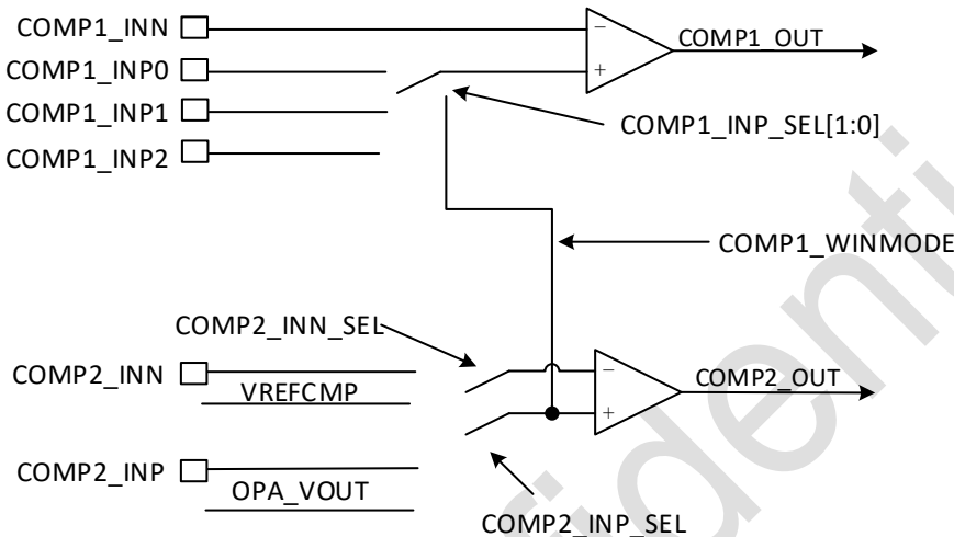
图 12-2 window 比较器
