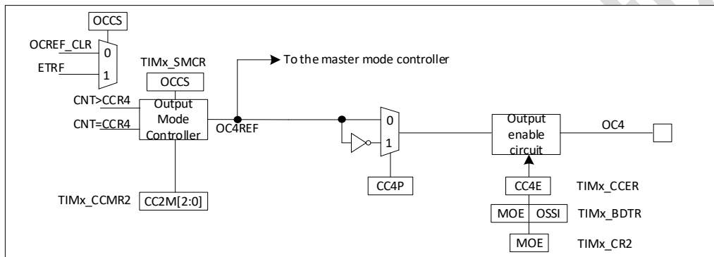
图 13-30 捕获/比较通道的输出部分(通道 4)
