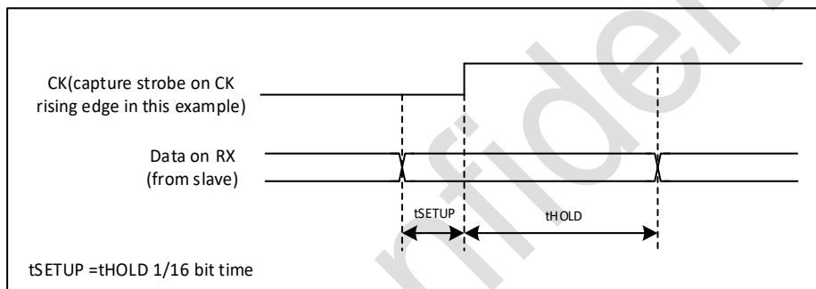
图 18-12 RX 数据建立/保持时间
