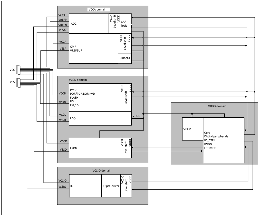
图 5-1 电源框图
