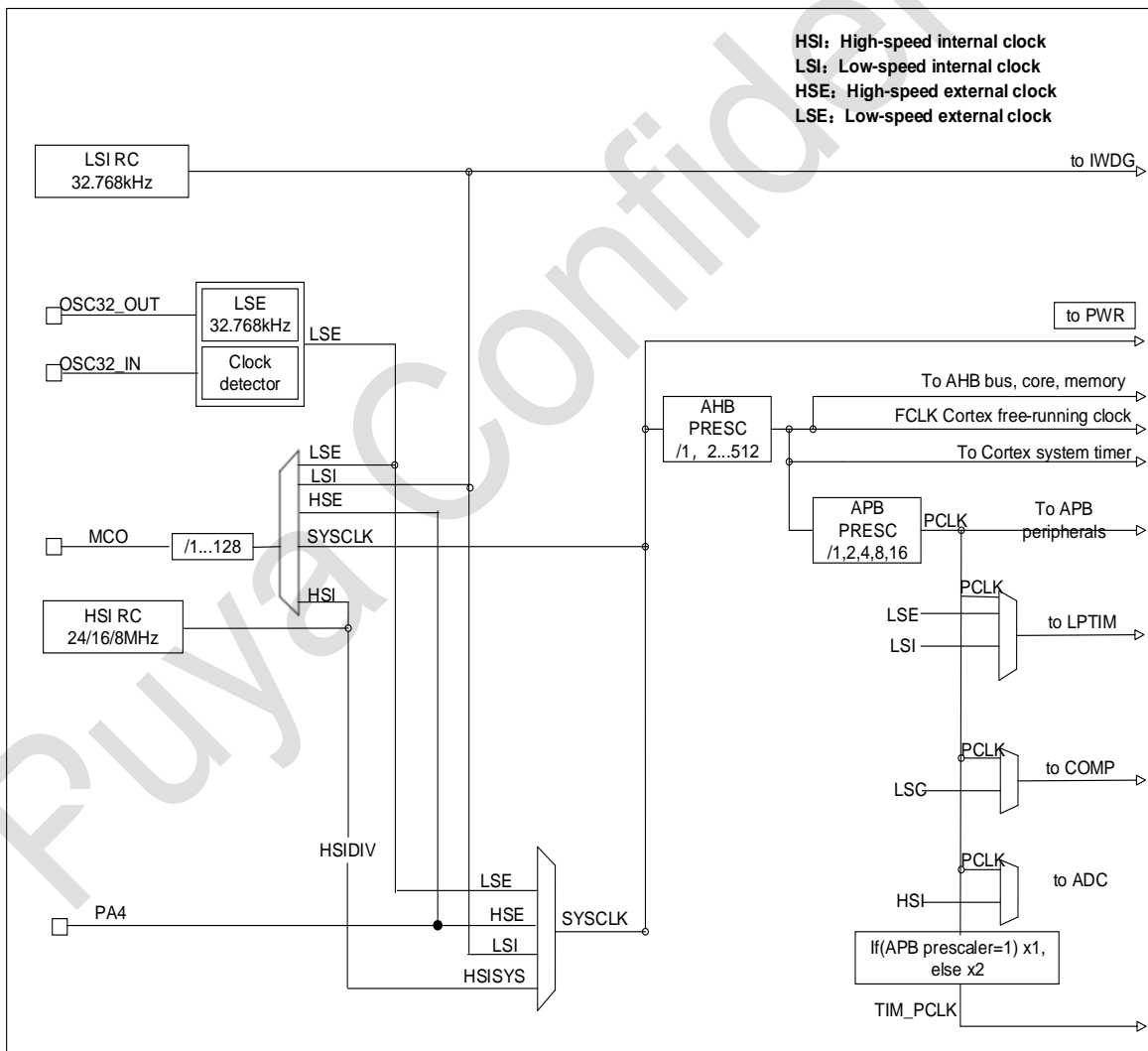
图 6-2 系统时钟结构图
