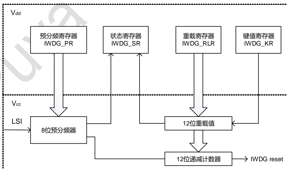
图 17-1 IWDG 框图
