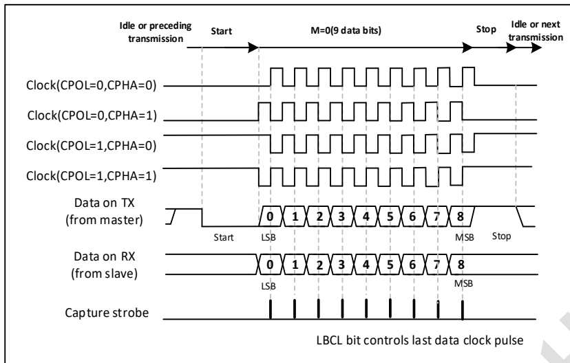
图 18-11 USART 数据时钟时序示例(M=1)
